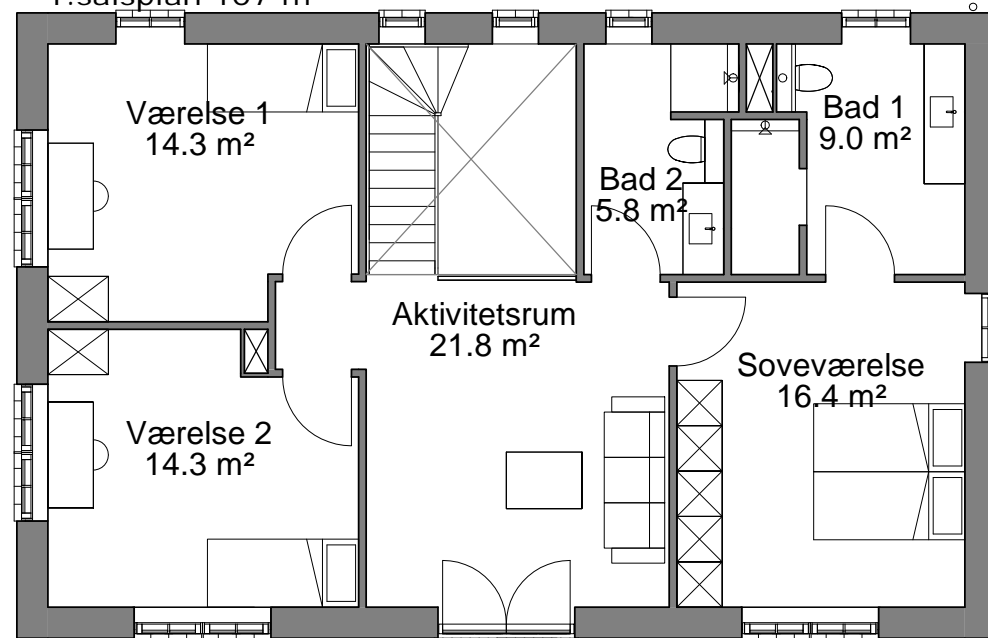
1.salsplan 107 m²
