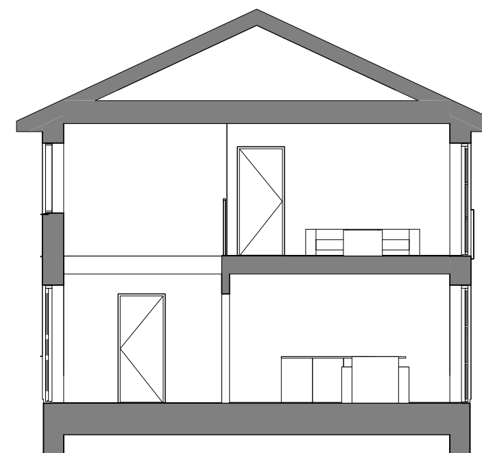
Principssnit
